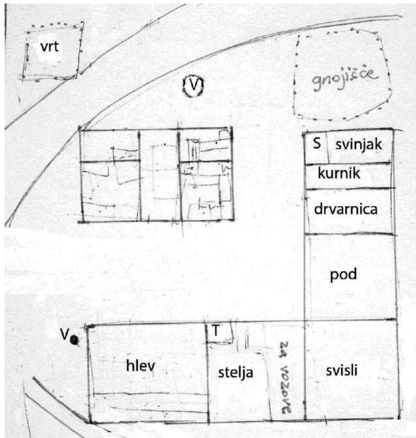
Skica 4: Tloris gospodarskega poslopja v času, ko je imelo še obliko črke L.
