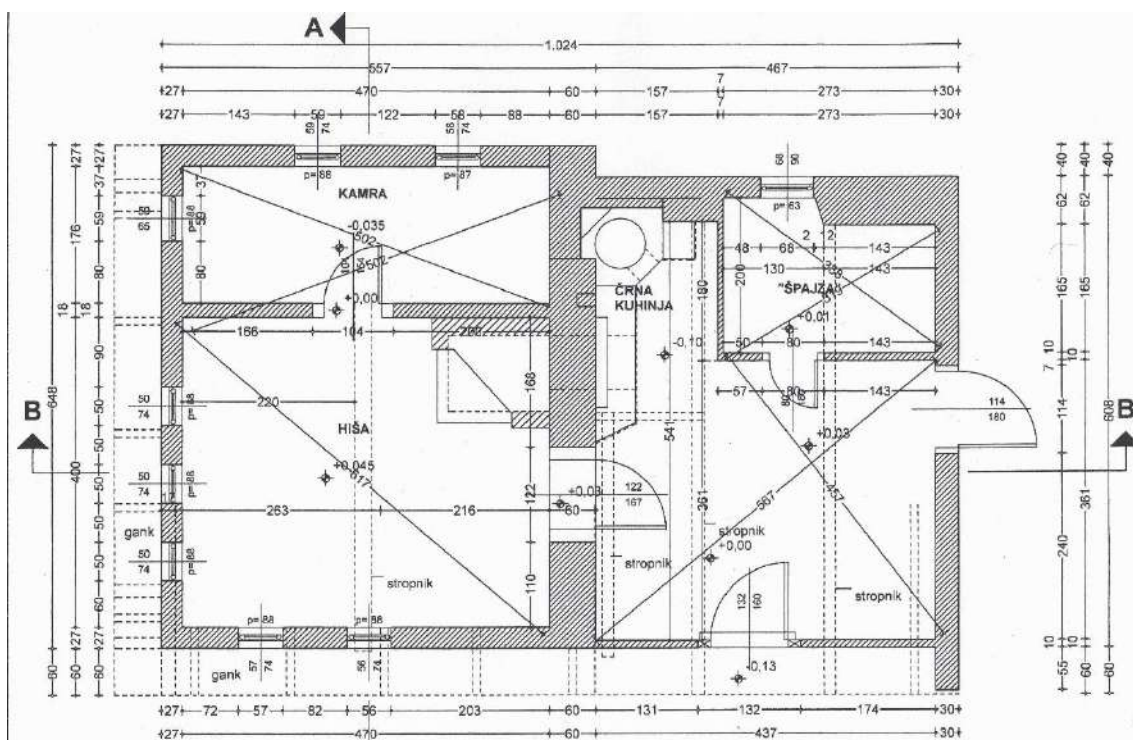
Skica 3: Tloris pritličja – konstrukcija, povzeto po projektni dokumentaciji Metric d. o. o. 32
