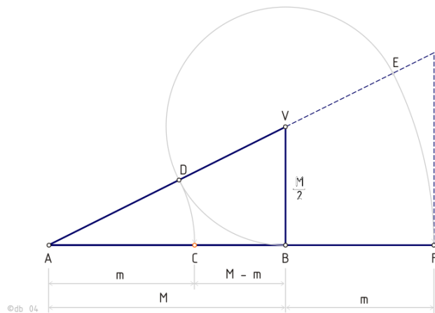
Slika 6: Konstrukcija zlate točke (vir: https://upload.wikimedia.org/wikipedia/sl/2/2b/Daljica_konst1.png )
