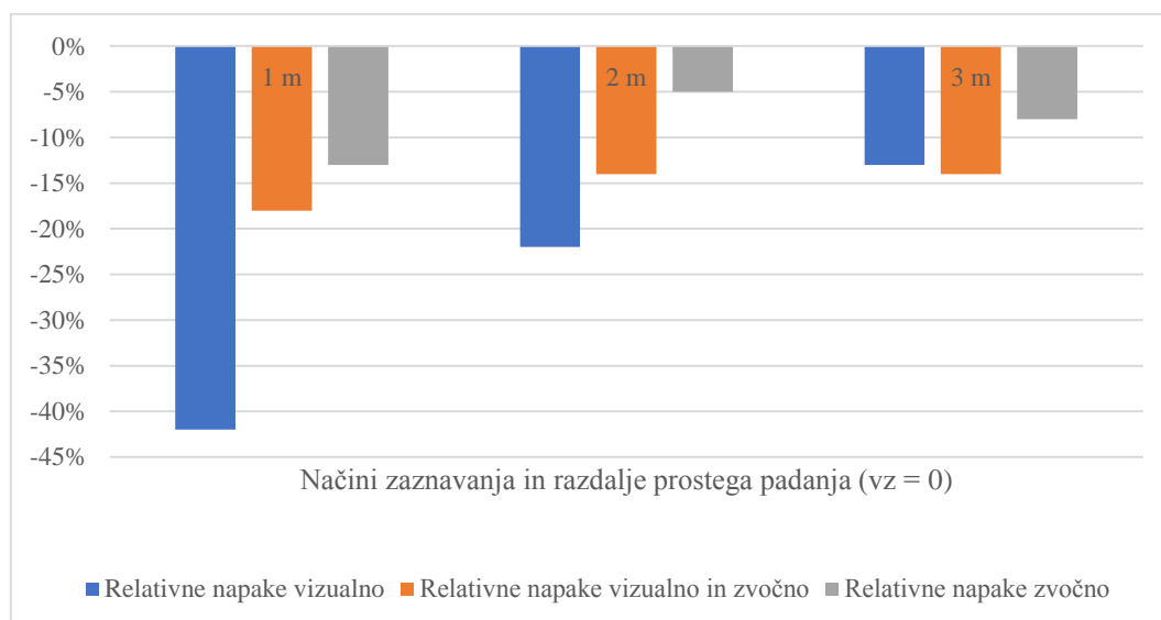
Grafikon 4 Primerjava povprečja relativnih napak meritev glede na način zaznavanja začetka in konca padanja kroglice (vir:avtorji)
