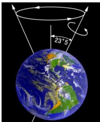
Slika 6: Nagnjenost Zemlje
