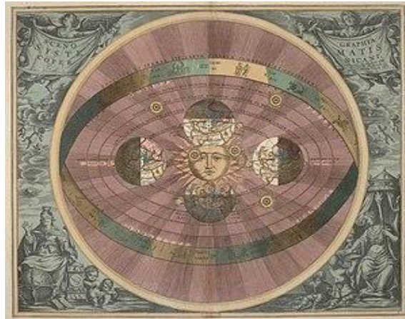
Slika 3: Heliocentrični sistem
