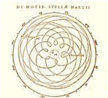
Slika 4: Geocentrični sistem
