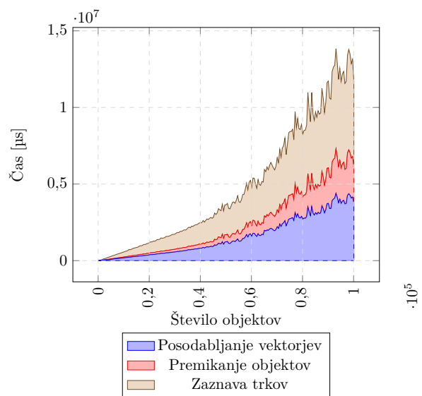
Slika 7: Vpliv števila objektov na hitrost simulatorja
