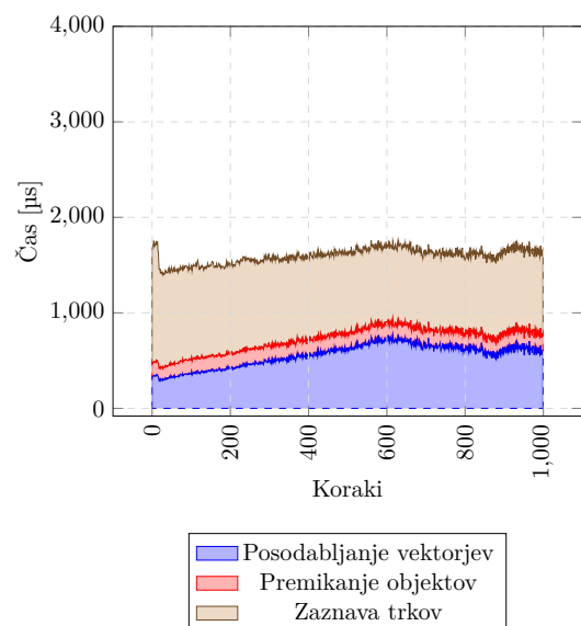
Slika 15: Vključena reciklaža in vključena gravitacija
