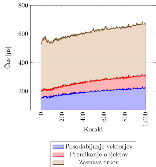
Slika 12: Vključena reciklaža in izključena gravitacija
