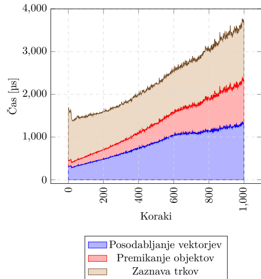
Slika 14: Izklopljena reciklaža in vklopljena gravitacija
