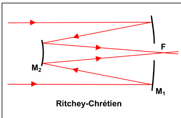
Slika 14: Primer poti svetlobnih žarkov skozi teleskop tipa Ritchey-Chrétien. Svetloba se najprej odbije od primarnega zrcala (M 1 ) in nato od sekundarnega (M 2 ) [vir: https://commons.wikimedia.org/wiki/File:Diagram_Reflector_RitcheyChrétien.svg ]
