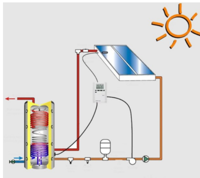
Slika 7: Solarni sistem
