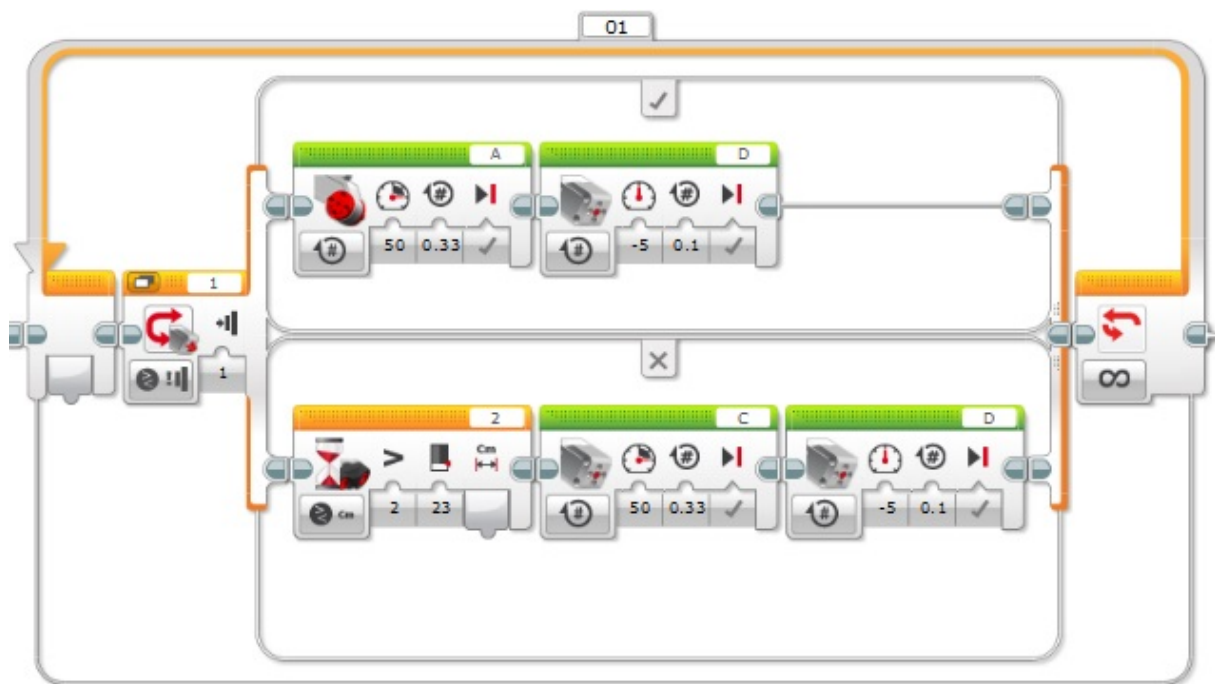
Slika 18: Program za peč in TČ (Foto: M. Meh)
