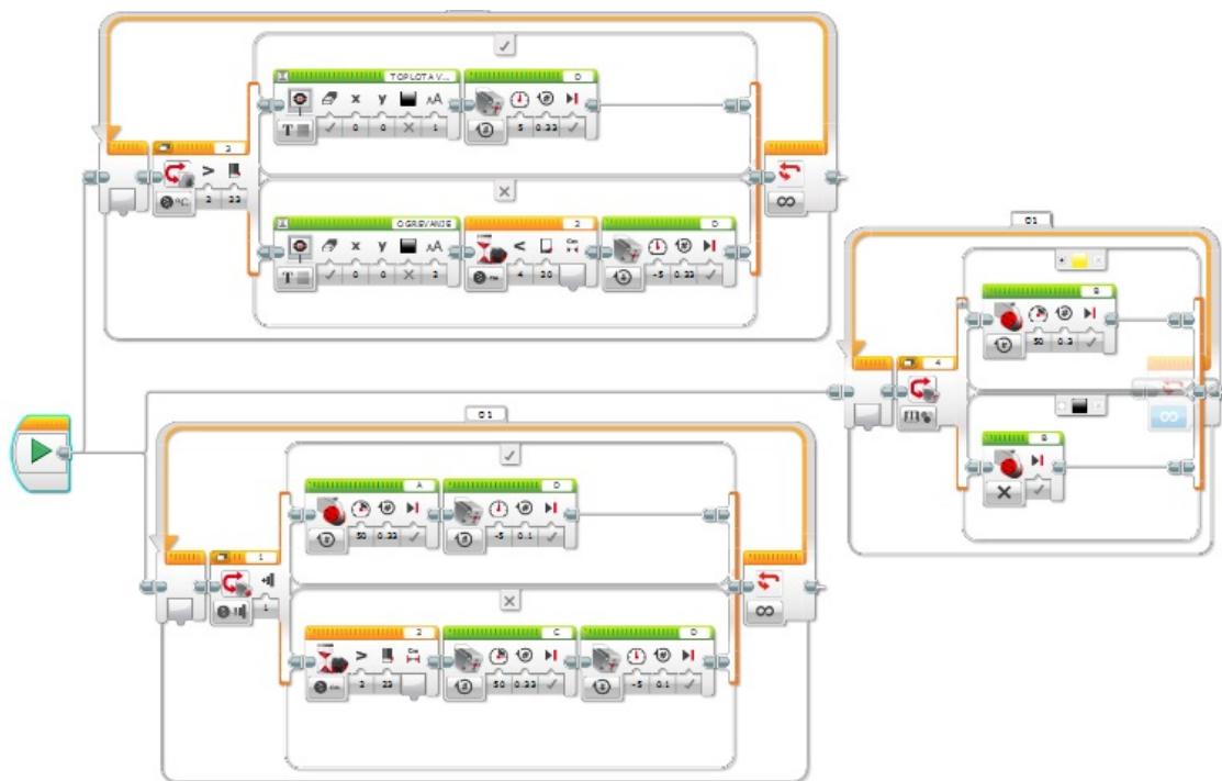
Slika 19: Celoten program (Foto: M. Meh)
