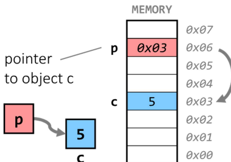
Slika 19: Kazalniki v pomnilniku [25]
