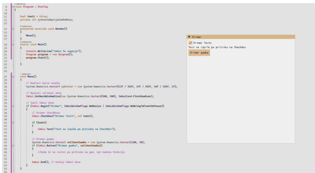
Slika 4: Uporaba Dear ImGui (vir: lasten)
