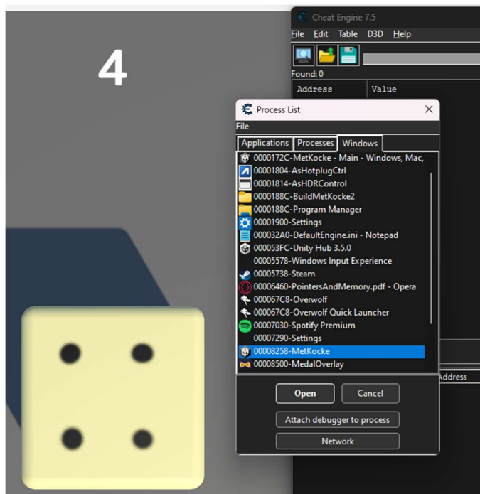
Slika 13: Izbiranje aplikacije za iskanje pomnilniških naslovov s programom Cheat Engine (vir: lasten)
