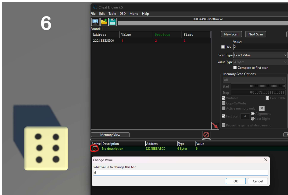
Slika 8: Spreminjanje vrednosti kocke v Cheat Enginu (vir: lasten)
