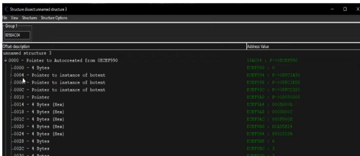
Slika 22: Cheat Engine pogled v pomnilnik (vir: lasten)
