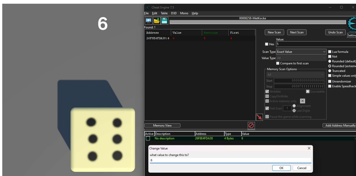
Slika 15: Nastavljanje vrednosti kocke v Cheat Engine (vir: lasten)
