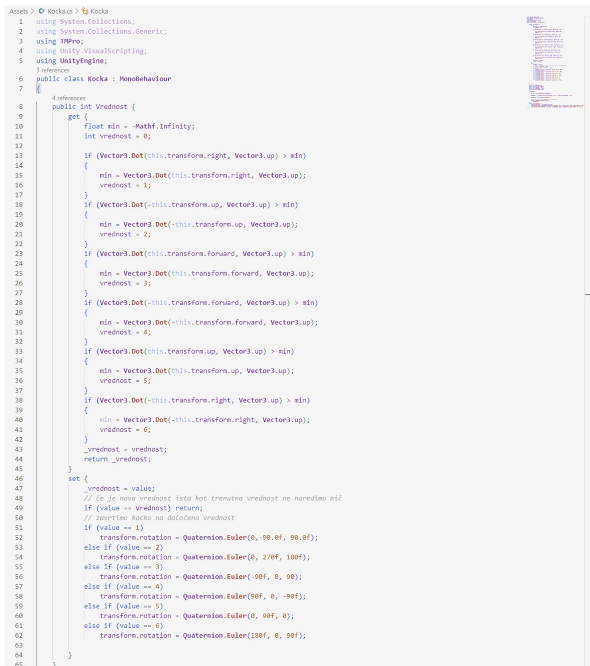
Slika 10: Koda za branje in nastavljanje rotacije kocke z metodama "set" in "get" (vir: lasten)
