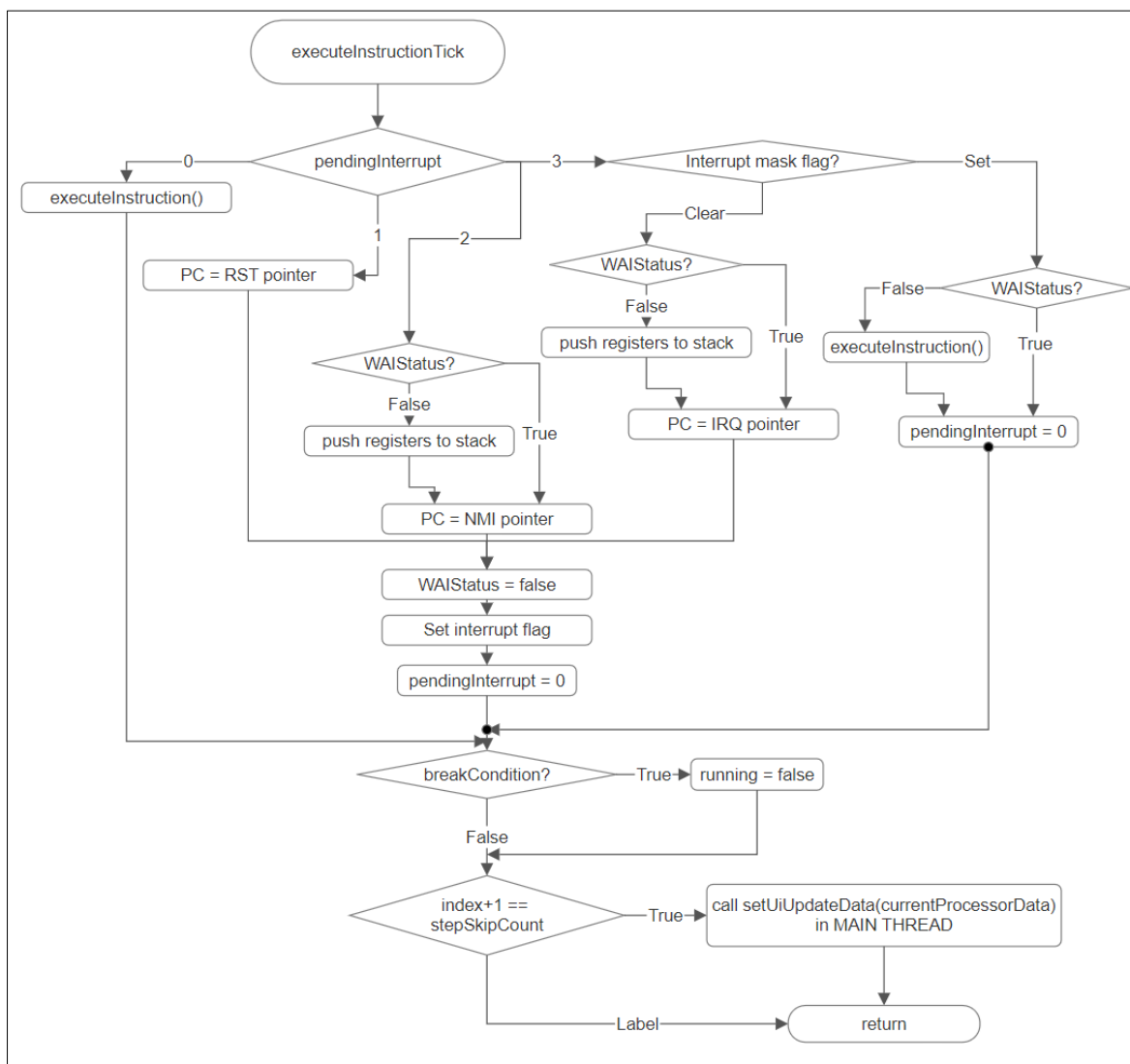
Slika 34: Diagram poteka: Funkcija startExecution: executeInstructionTick (vir: lasten vir)
