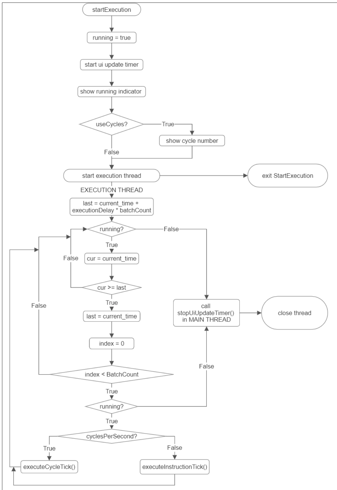
Slika 32: Diagram poteka: Funkcija StartExecution (vir: lasten vir)
