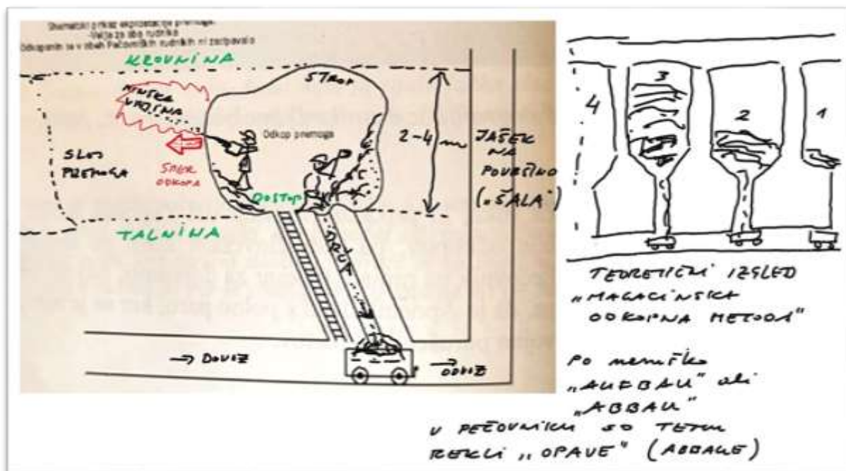
Slika 87: Metoda odkopavanja premoga v Pečovniku. Vir: Bobnič, 2012. Dopolnjeno z detajli dr. Salobir, 2024.
