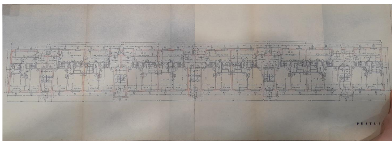
Slika 59: Tloris bloka tipa i (SI_ZAL_LJU t. e. 354 p. e. 26).
