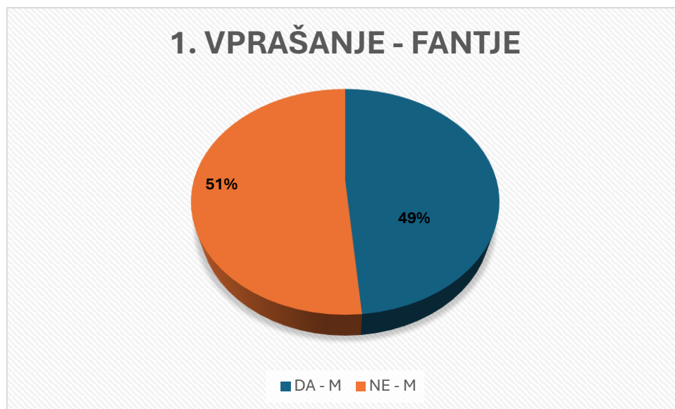
Graf 4: Odgovori fantov na prvo vprašanje
