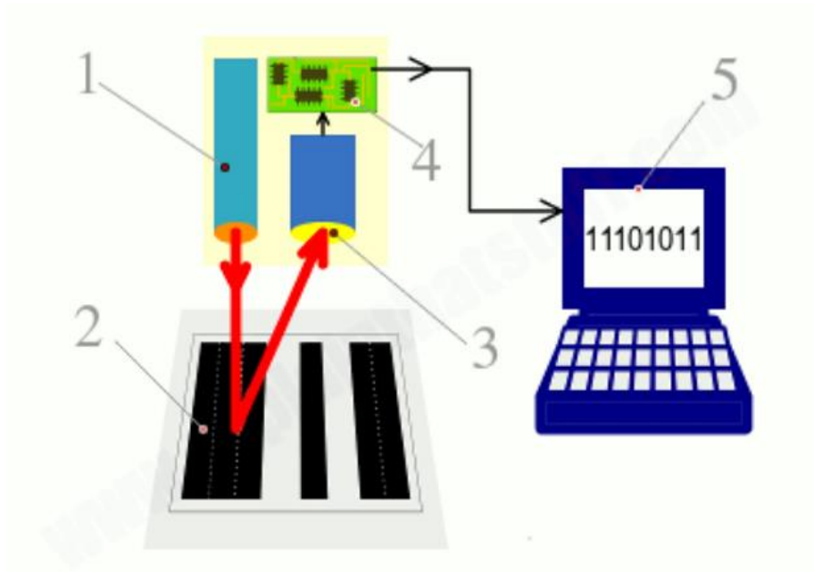
Slika 6: Čitalnik kode.
