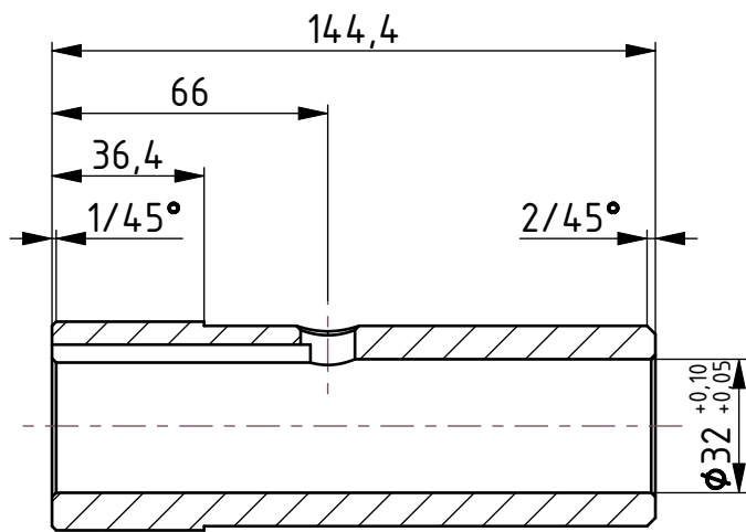
Prerez A-A
