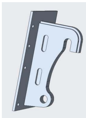
Slika 39: Idejni model priklopne plošče z vpetjem Atlas (Osebni vir)
