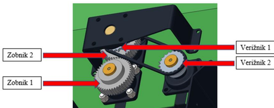
Slika 30: Zobniški in verižni prenos vrtenja
