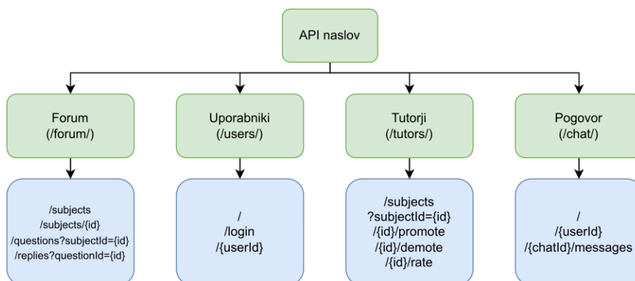
Slika 154: Končne točke najinega spletnega vmesnika (lasten vir)
