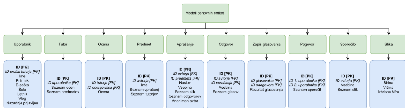
Slika 155: Diagram definicij razredov osnovnih entitet za shranjevanje v podatkovni bazi (lasten vir) (PK – primarni ključ, FK – tuji ključ)
