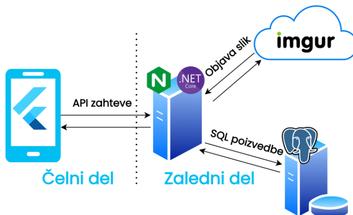
Slika 1: Shema arhitekture najine aplikacije (lasten vir, ustvarjena s spletnim orodjem Diagrams.net)
