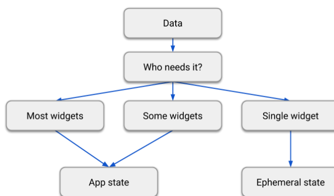
Slika 75: Delitev na aplikacijsko in kratkotrajno stanje [39]
