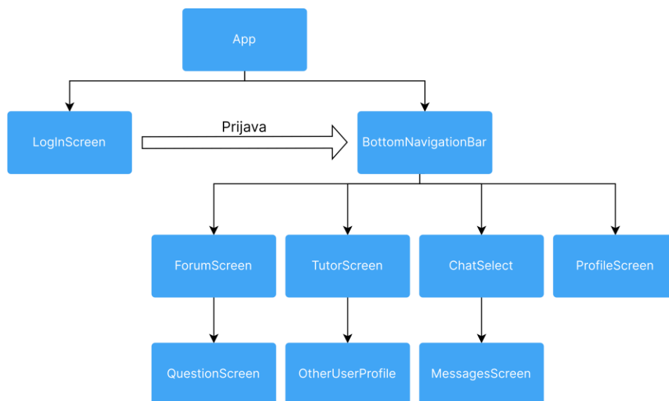
Slika 153: Osnovna struktura gradnikov mobilne aplikacije (lasten vir)
