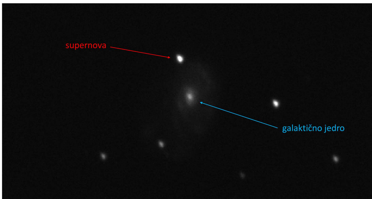
Slika 5: Približan posnetek supernove z galaksijo v kateri je eksplodirala v modrem filtru
