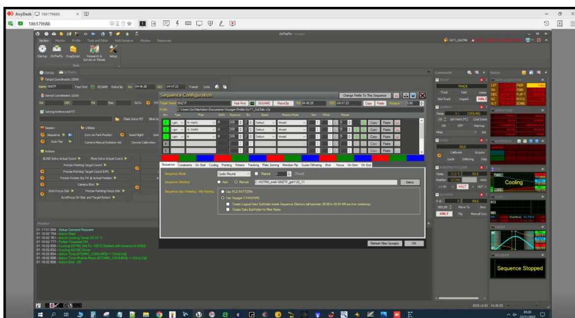
Slika 3: Posnetek zaslona iz programa Voyager
