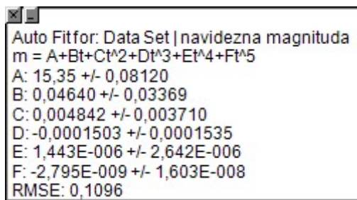
Slika 9: Podatki za predpis za prilagoditveno krivuljo v programu Logger Pro
