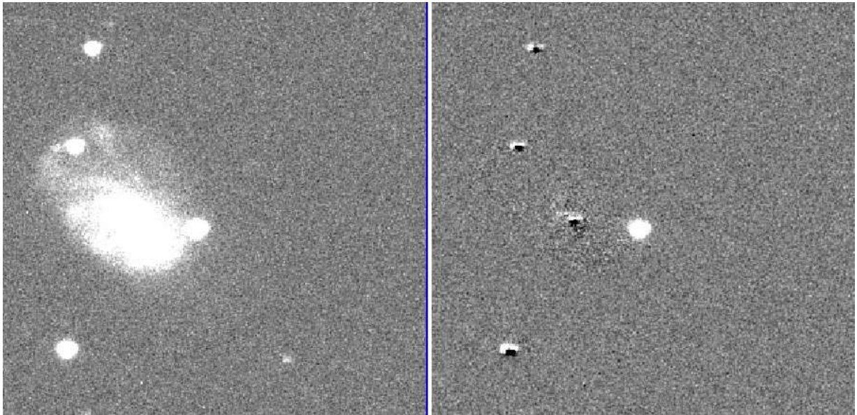
Slika 7: Fotografija supernove pred odšteti galaksije in po njem
