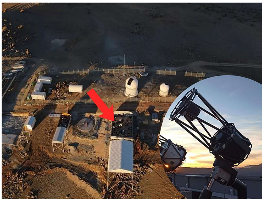
Slika 2: Teleskop GoT1 in njegova lokacija ( https://www.gochile.si/ )
