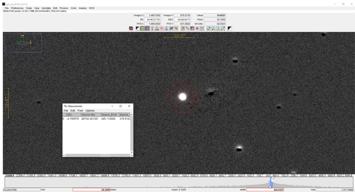
Slika 8: Posnetek zaslona iz programa AstroImageJ
