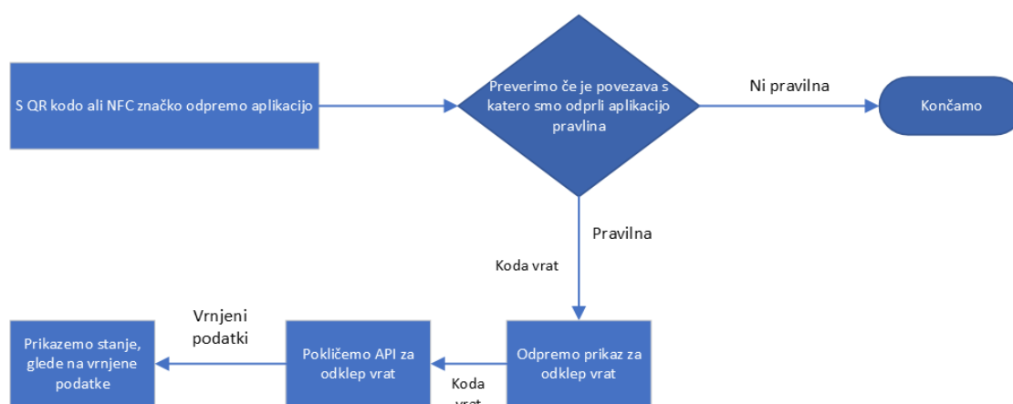
Slika 29: Prikazuje diagram poteke za delovanje mobilne aplikacije (Vir: lasten)
