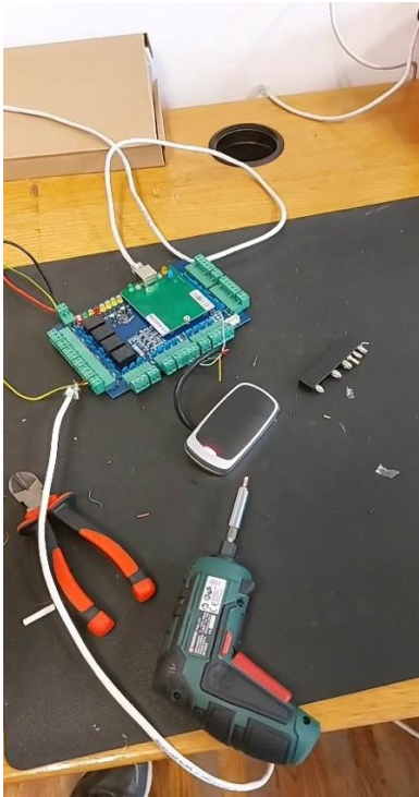
Slika 2: Prototip priklopa čitalnika na krmilnik (Vir: lasten)
