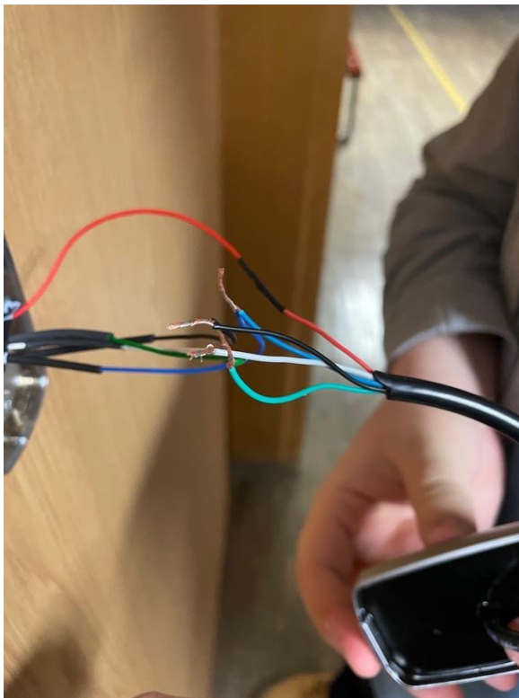
Slika 9: Nameščanje bralnika kartic na zunanja vrata kabineta (Vir: lasten)
