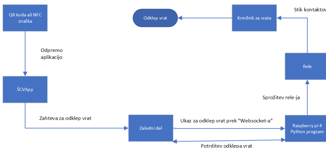
Slika 31: Prikazuje diagram poteka za celoten sistem za odklep vrat preko aplikacije. (Vir: lasten)
