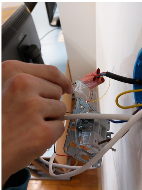
Slika 6: Spajanje kablov (Vir: lasten)
