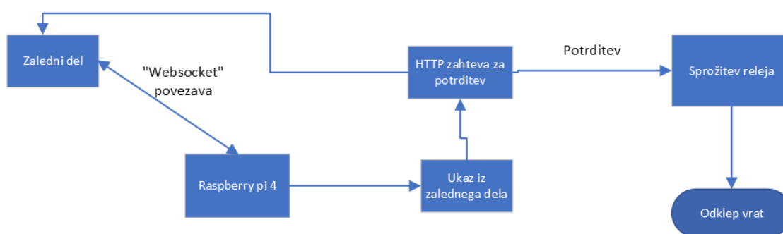
Slika 30: Prikazuje diagram poteka za delovanje Raspberry pi 4 (Vir: lasten)
