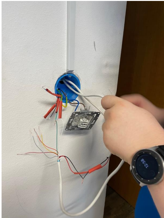
Slika 5: Priprava na spajanje kablov (Vir: lasten)
