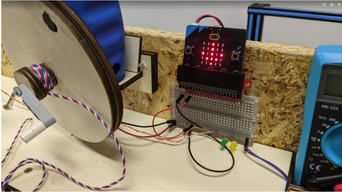
Slika 9: Dodali smo Micro:bit, ki računa, koliko energije proizvedemo. (Fotografija: Lina Ledinek)
