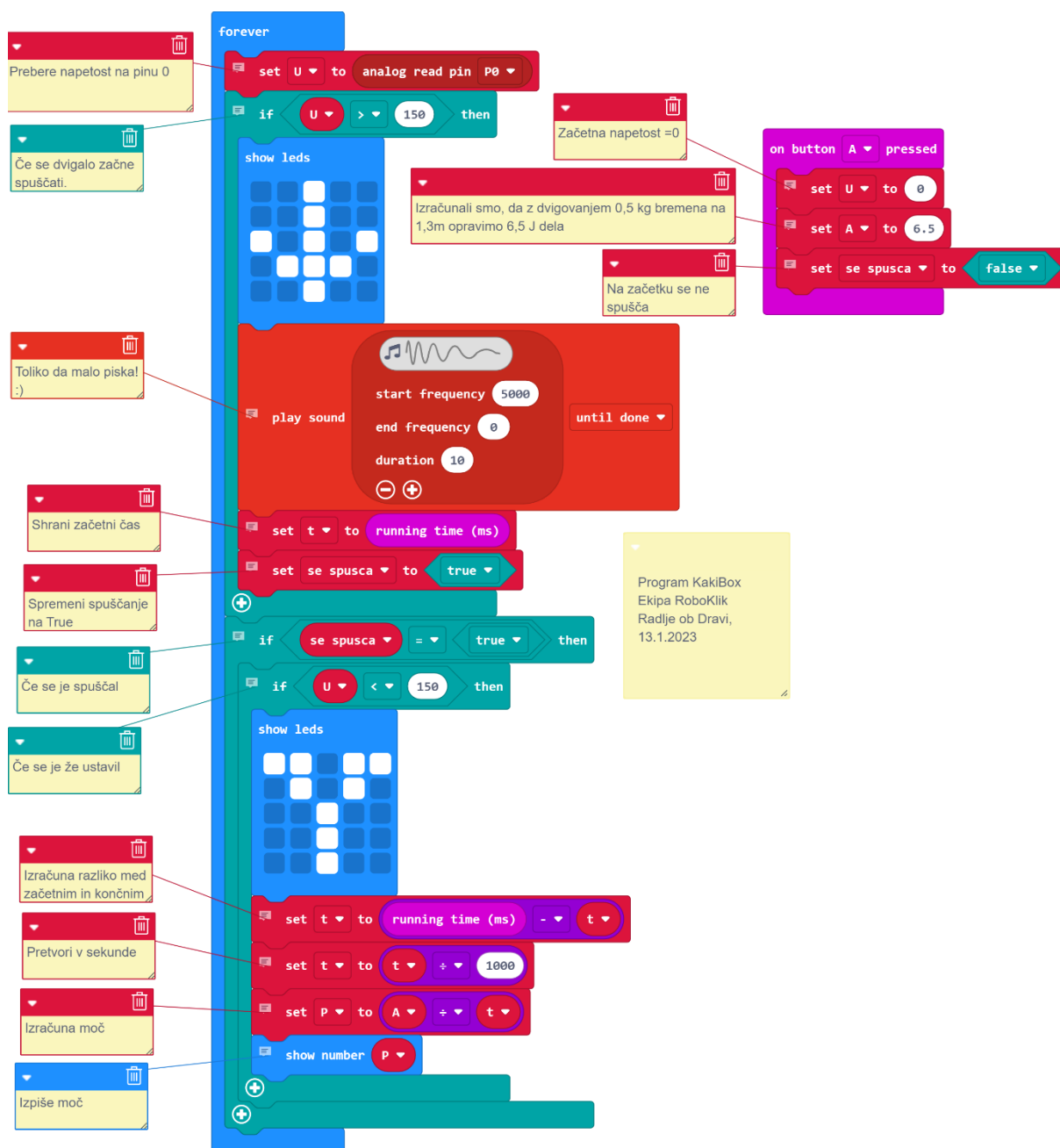
Slika 25: Naš model smo nadgradili z Micro:bitom, ki računa izhodno moč. (Avtor: Alex Glazer in Špela Škorjanc)
