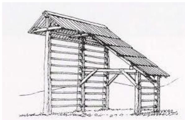
Slika 7: Enojni kozolec z nadstreškom
