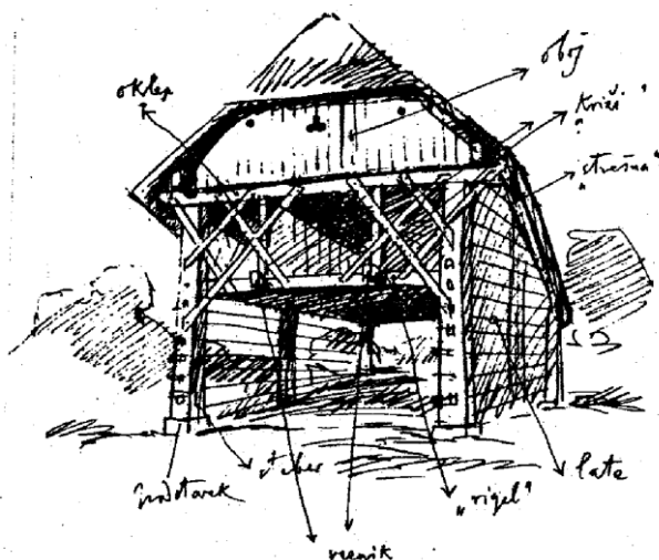
Slika 3: Sestavni deli kozolca
